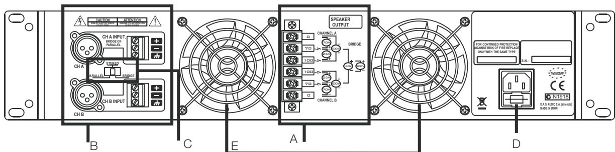
Detalle de las entradas XLR y Terminal Block
