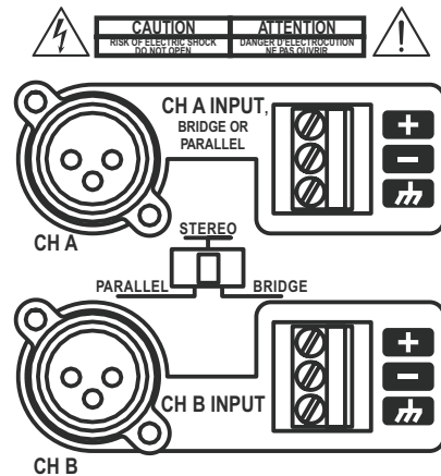
Detalle de las entradas XLR y Terminal Block
